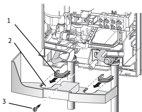
Instrucciones de montaje para grifería "vista" (AP)
