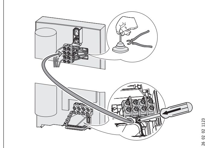
Conexión eléctrica arriba
