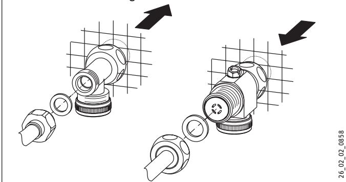
Toma de conexión de agua
