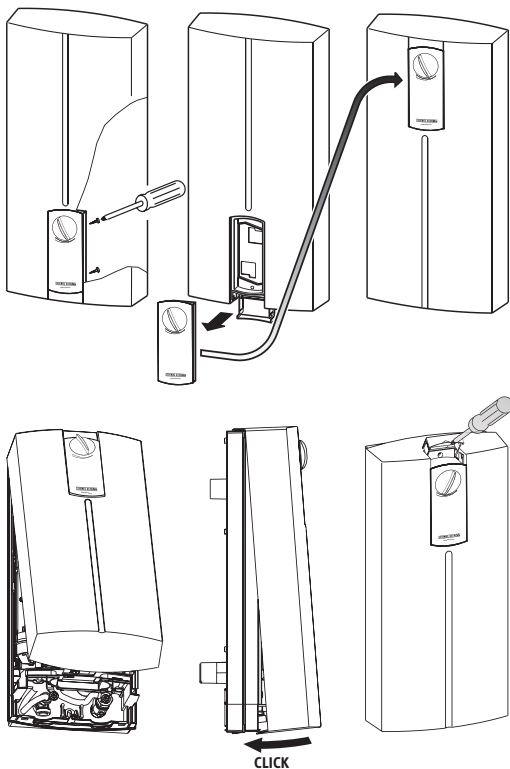
Tapa del equipo con montaje bajo una mesa
