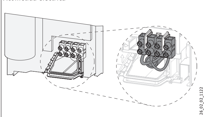
Acometida eléctrica
