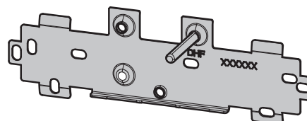
Barra de enganche con sustitución de equipo DHF
