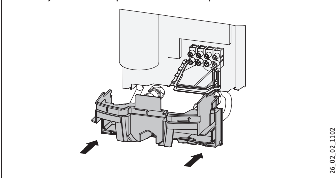
Montar y enclavar la parte inferior del panel trasero
