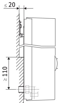
Dim. de instalación en los espacios o juntas entre baldosines
